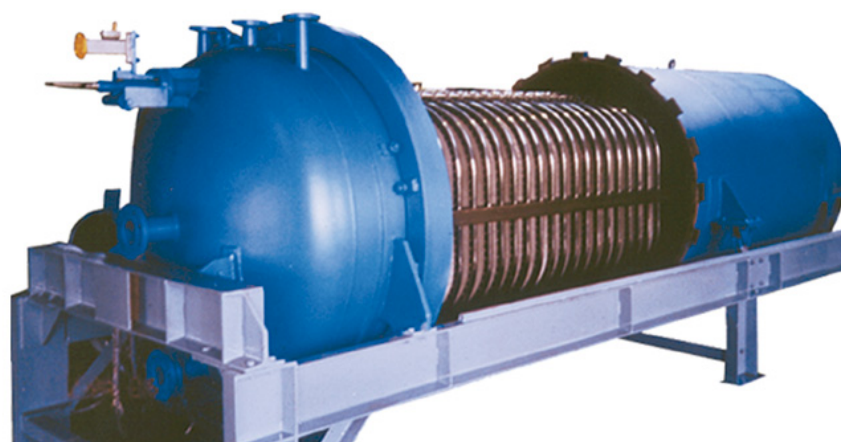
* Filtro de Placas Horizontales para filtración de ceras en planta de aceite comestible.
